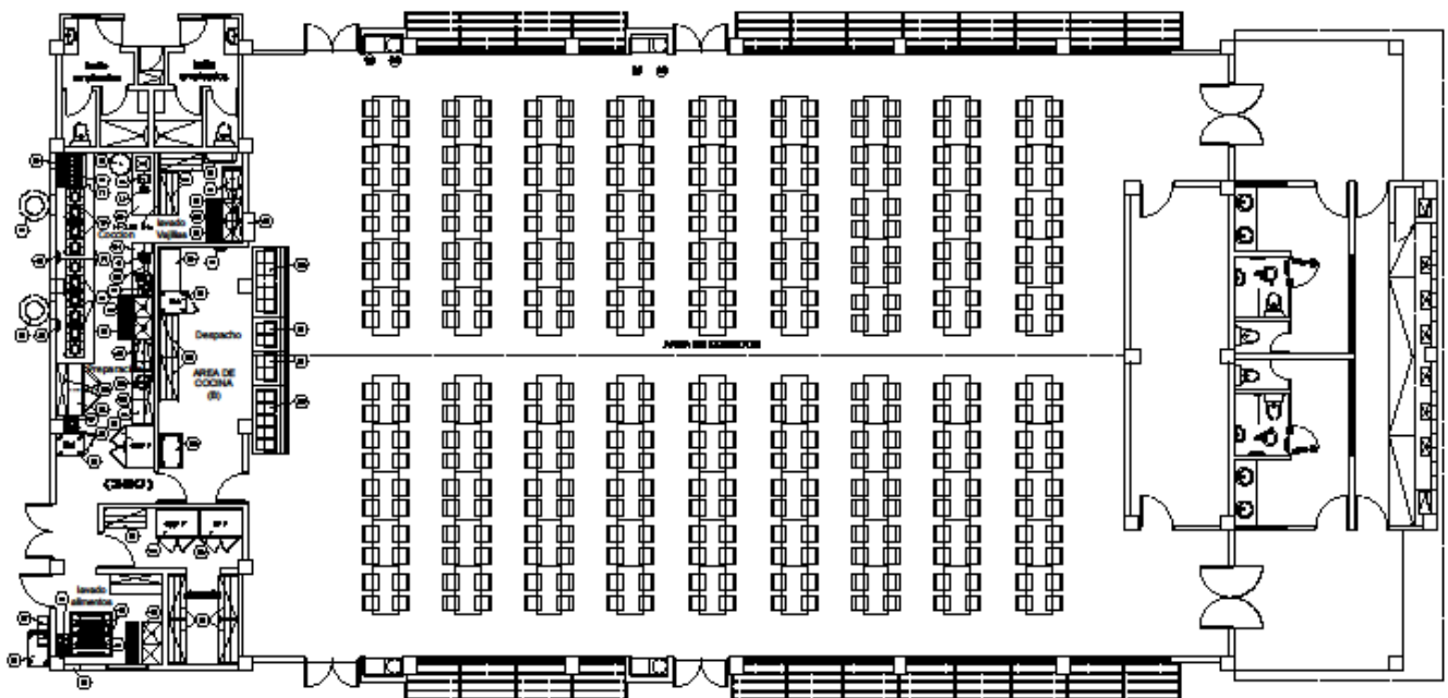
1 A1 PLANTA AMUEBLADA COCINA-COMEDOR 360 ESTUDIANTES ESC.:1:75
