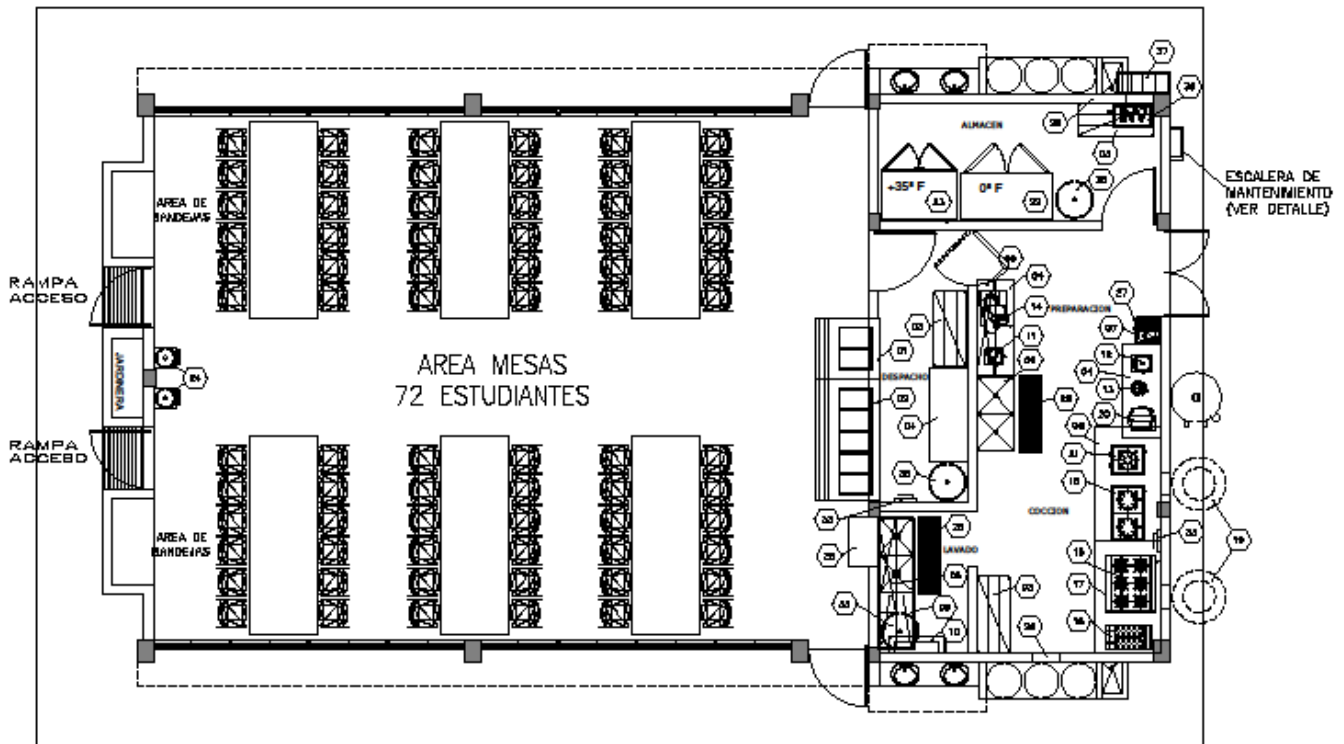
PLANTA AMUEBLADA COCINA-COMEDOR TIPO "B" (72 PERSONAS)
